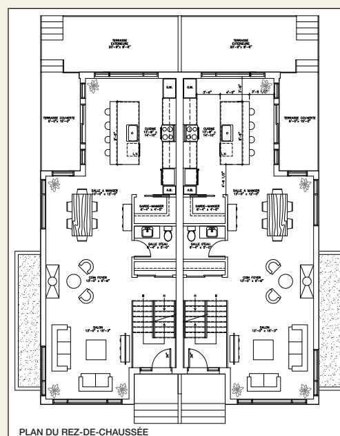
PLAN DU REZ-DE-CHAUSSEE
