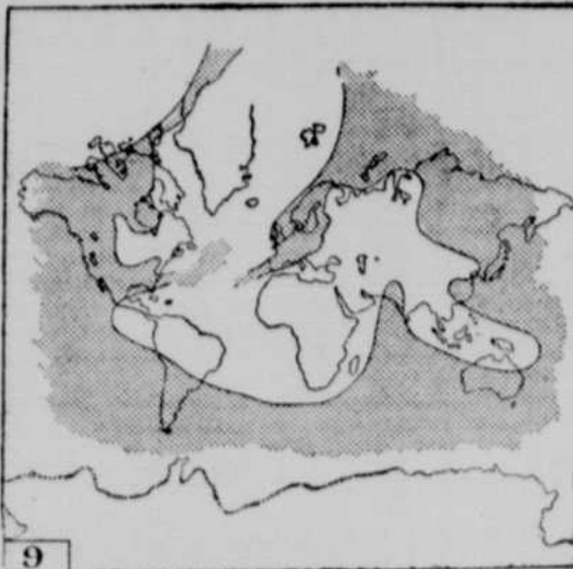
LES PREMIERES TERRES EMERGÉES
