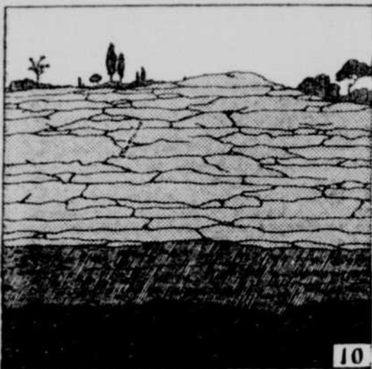
LA STRATIFICATION DE L'ECORCE TERRESTRE
