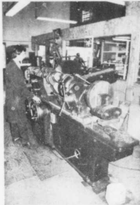
Un appareil impressionnant une rectifieuse de vilebrequins pour réusinier avec rayons les vilebrequins. Il s'agit, ici, d'un vilebrequin de marque Caterpillar confié aux soins de Robert Pro-novost. Toutes les autres marques re-çoivent la même attention experte.
