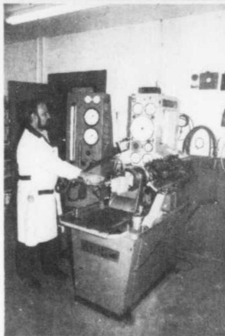
Réjean Lemieux s'affaire ici au délicat travail d'équilibrage d'une pompe, dans le cas présent, une pompe de marque Cummins. Un autre exemple de l'outillage moderne et précis de Système Injection La Mauricie Inc.
