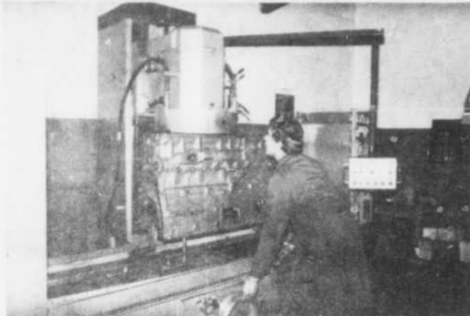
Sur la photo ci-haut, nous apercevons Sylvain Laffeur à l'oeuvre sur une machine de précision servant à planer les moteurs. Ici, il s'agit d'un moteur Cummins. Un outillage nouveau et automatique pour des résultats parfaits.
