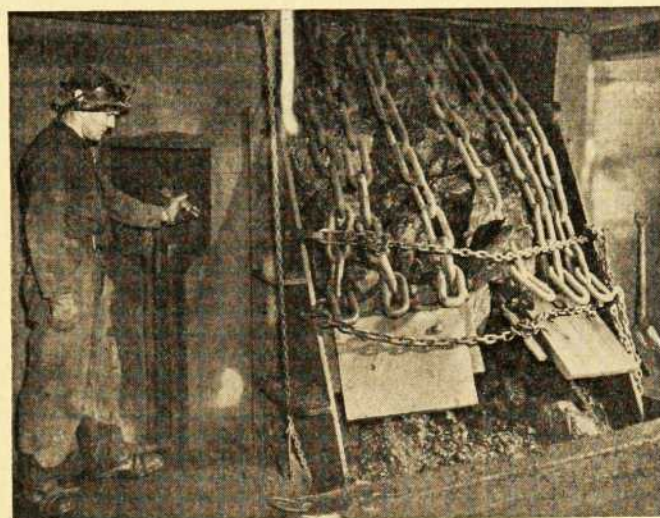
La "bouche" d'une concasseuse à minerai qui est prévue pour emplir les camions d'un seul coup et presque sans interruption.
