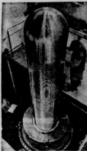
● RESSEMBLANT à un projectile téléguidé tout rutilant, cet appareil est en réalité un générateur électrostatique au centre de recherches atomiques d'Aldermaston, en Angleterre. Il peut produire six millions de volts d'électricité.
