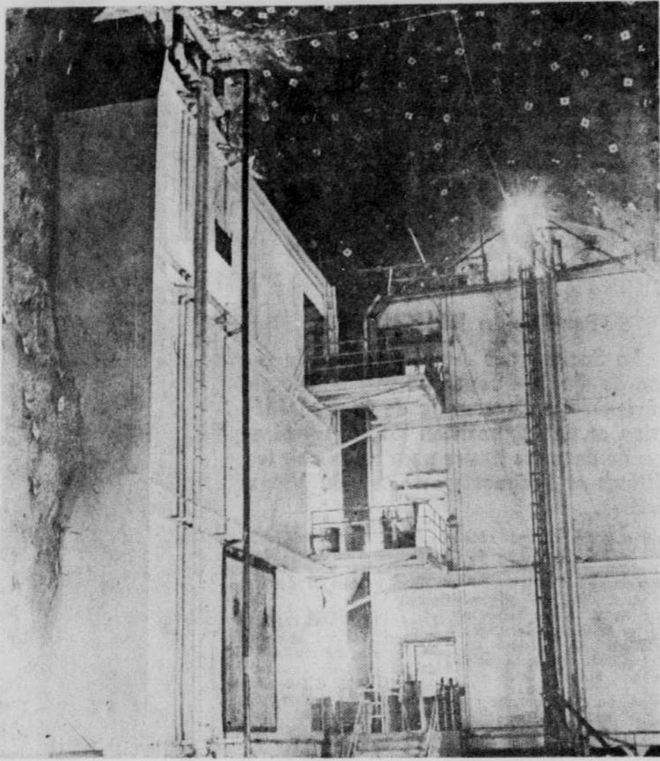
EN ACIER SOUS UN DOME DE GRANIT — Voici deux des onze édifices en acier du centre de commandement de défense aérienne de l'Amérique du Nord. L'intérieur
