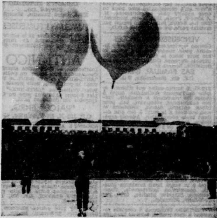
CES BALLONS lancés par des savants de l'université de Chicago portaient des appareils destinés à enregistrer un orage de rayons cosmiques déterminé par une explosion de gaz dont la force équivalait à celle d'un million de bombes hydrogènes.
