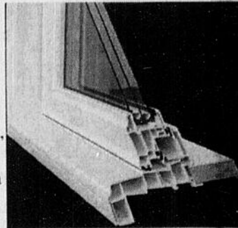
Coupe de fenêtre Série Prestige HT-1000.
