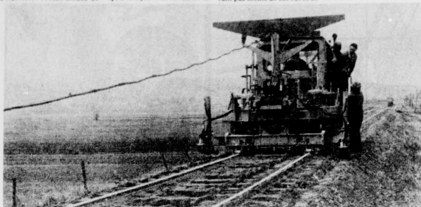
SUITE D'INONDATION — La compagnie ferroviaire Québec Central exécute des travaux importants pour rétablir le niveau de la voie ferrée, entre les villes de Saint-Joseph et de Vallée-Jonction, dans Beauce-Nord.
