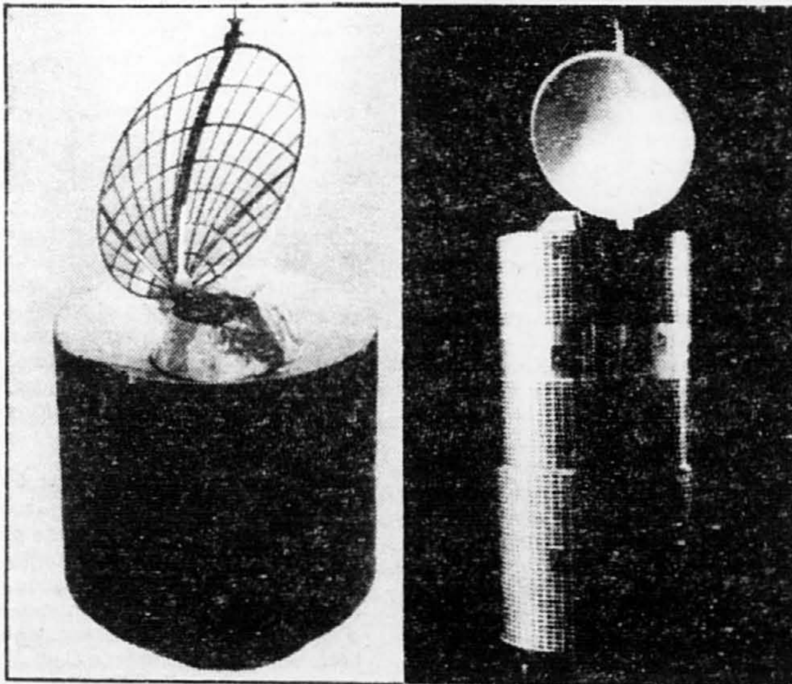
À gauche, l'Anik-1, premier satellite de télécommunication au monde mis sur orbite géostationnaire (1972); à droite, l'Anik C-1 lancé en 1982 pour assurer la radio-télédiffusion et la télé payante pour une autre décennie.
