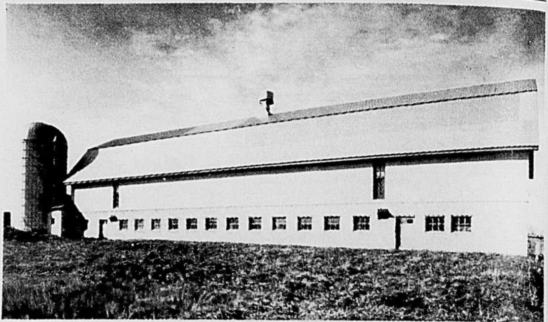
Grange à l'épreuve du feu, entièrement en béton, située près de Dorion, P.Q. On notera l'utilisation combinée des panneaux de béton et de la maçonnerie de béton. Silo en dômes de béton.
