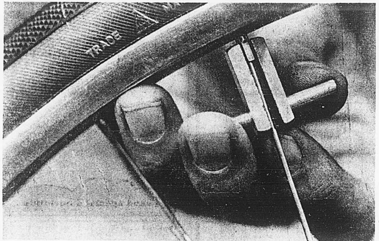
Resserrer ou desserrer la douille-écrou du rayon pour augmenter ou diminuer la tension de celui-ci.
