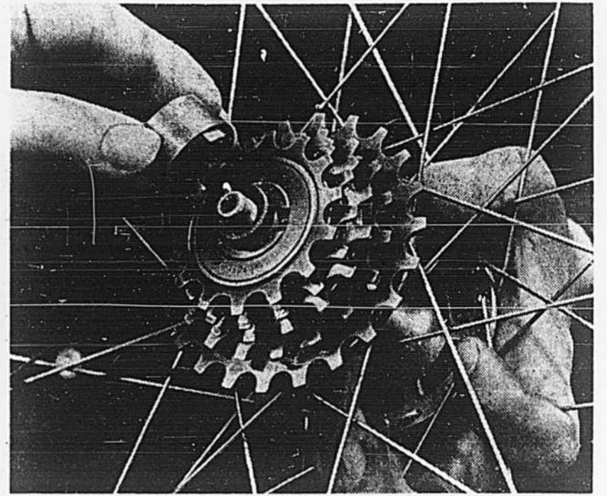
Pour détacher l'ensemble des pignons de la roue, il existe une clé spéciale ayant la forme d'un barillet que le démonstrateur tient entre ses doigts.
