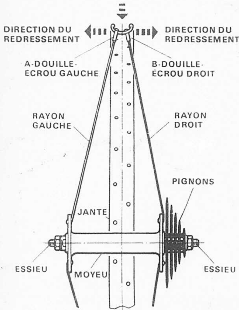
LE REDRESSEMENT DE LA JANTE
