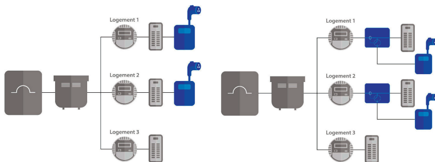
Figure 1 – Solutions individuelles sur le panneau et l'artère du logement
