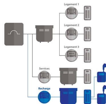
Figure 2 – Solution partagée avec un branchement dédié à la recharge de VÉ
