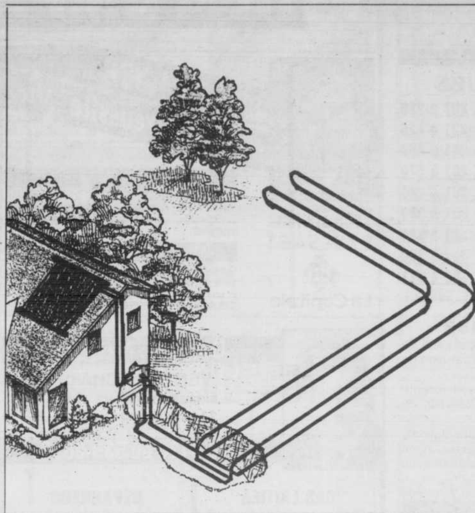
Couplage d'un chauffe-eau solaire à une pompe géothermique pour une efficacité optimum.
