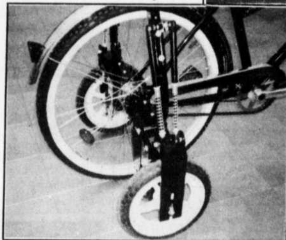
Le BY-O est un kit de transformation unique pour convertir un vélo en tricycle.
