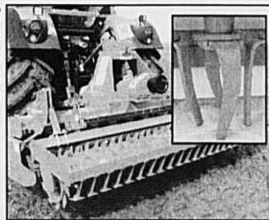
NGH NGS Herse rotative (de 3 à 4.5 mètres avec des dents agressives)
