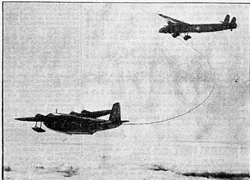
En vue de l'établissement de services transatlantiques réguliers, les Imperial Airways procèdent à de multiples expériences notamment celle du ravitaillement en plein vol. On voit sur cette photo l'hydravion Cabot recevant d'un autre avion une provision de 1,000 gallons d'essence sans pour cela interrompre son envolée.
