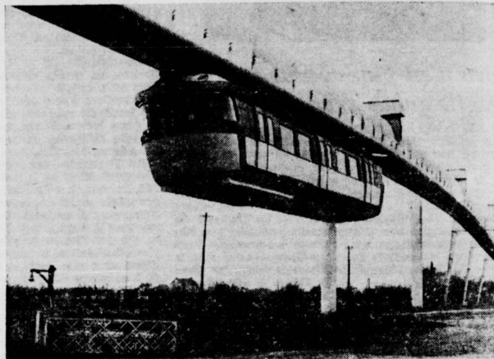
Le métro suspendu sur le parcours de démonstration de Châteauneuf-sur-Loire
