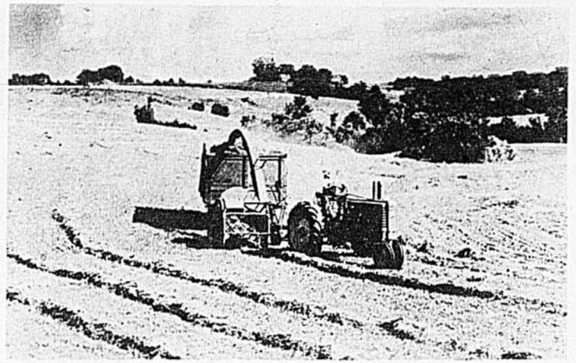
Avec ce type-ci, le foin doit d'abord avoir été fauché et mis en andains, ce qui demande nécessairement plus de main-d'oeuvre. Cependant, le foin peut être fané jusqu'au degré d'humidité idéal. Cette machine peut aussi servir à l'ensilage du maïs car on peut y adapter une "table à blé d'Inde".
