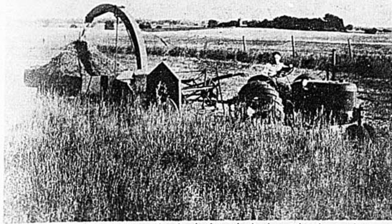
Voici le "coupe-fourrage" qui fauche le foin, le hache et le charge dans une seule et même opération. Un seul homme peut ainsi "faire ses foins" mais, pour un travail plus rapide, on aura deux autres wagons ; un deuxième homme fera le charroyage tandis qu'un troisième verra au déchargement.
