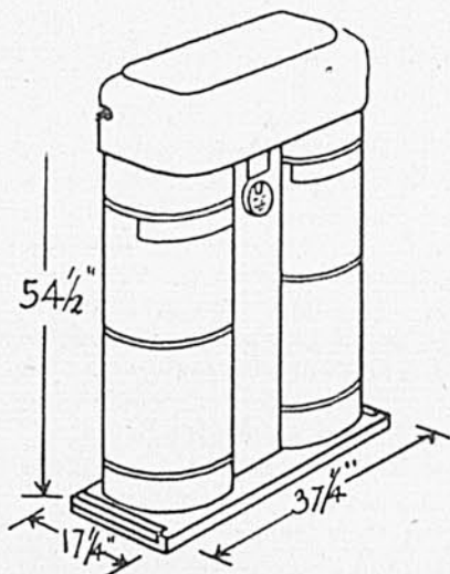
Deux genres d'installation à l'extérieur. A gauche, les cylindres sont placés dans un cabinet ou armoire. A droite, deux cylindres surmontés d'un couvercle double.
