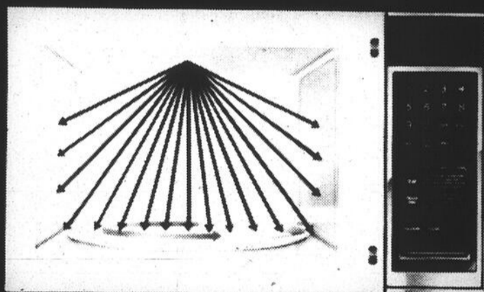
Trajet simulé des micro-ondes à leur entrée dans la plupart des fours à micro-ondes existants.
