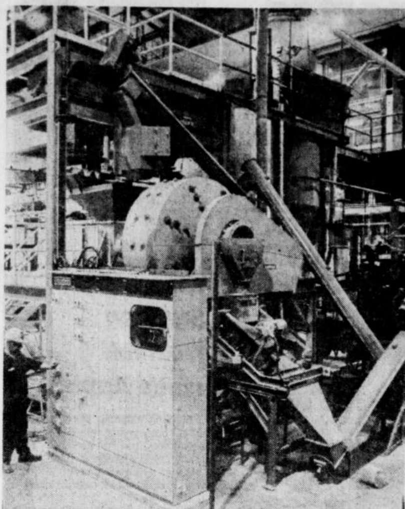
Les techniques de broyage du minerai sont mises à l'essai au Centre de recherches minérales à Québec dans ce broyeur autogène de l'usine pilote.
