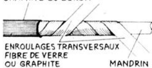
FIBRES LONGITUDINALES GRAPHITE OU BORON
