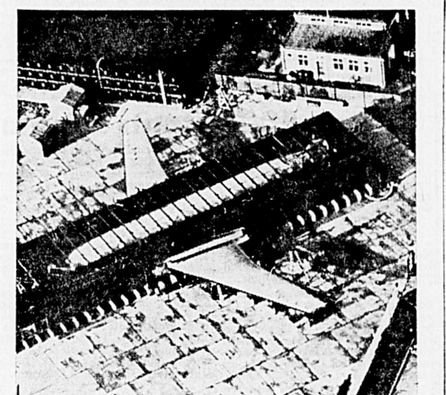
RESERVOIRS D'EAU AILES. — Cette photo donne une idée de l'énorme réservoir construit récemment par la compagnie de Havilland, à Hatfield, Grande-Bretagne, pour la vérification du fuselage des avions qu'elle manufacture. On voit ci-dessus les ailes d'un Comet II que le réservoir contient. Ce genre d'épreuve permet de se rendre compte de la résistance des appareils en plein air. Le réservoir a 140 pieds de long, 20 pieds de large et 16 de profondeur. Il contient 290,000 gallons d'eau. (CPC).
