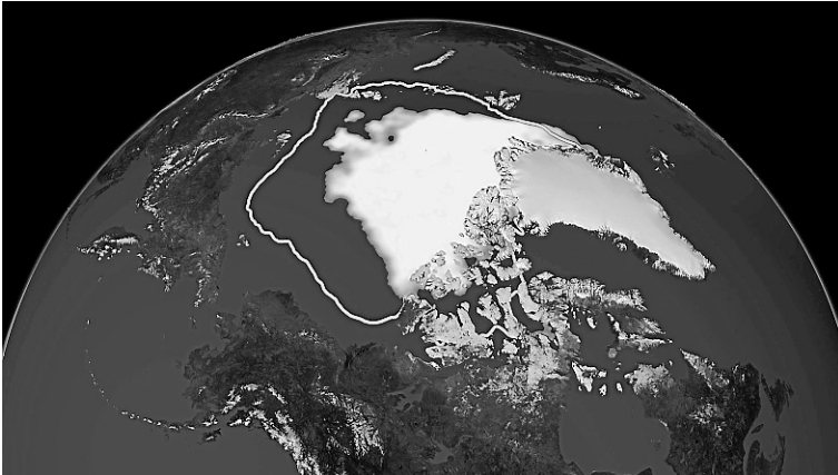
PHOTO ASSOCIATED PRESS Cette année, la banquise arctique a atteint sa plus faible superficie jamais observée: 3,4 millions de kilomètres carrés. C'est 700 000 km 2 de moins que le record précédent, établi en 2007 – l'équivalent de l'Alberta ou du Texas en moins.
