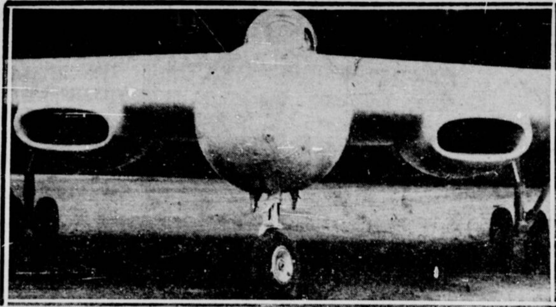
Voici une photographie du premier avion à fusée britannique, le A. W. 52, d'Armstrong Whitworth. Il est muni de deux turbopropulseurs Rolls Royce Derwent. Son aile a une envergure de 90 pieds. Comme on peut le voir, l'avion présente le minimum de résistance à l'air; c'est presque seulement une aile d'avion.
