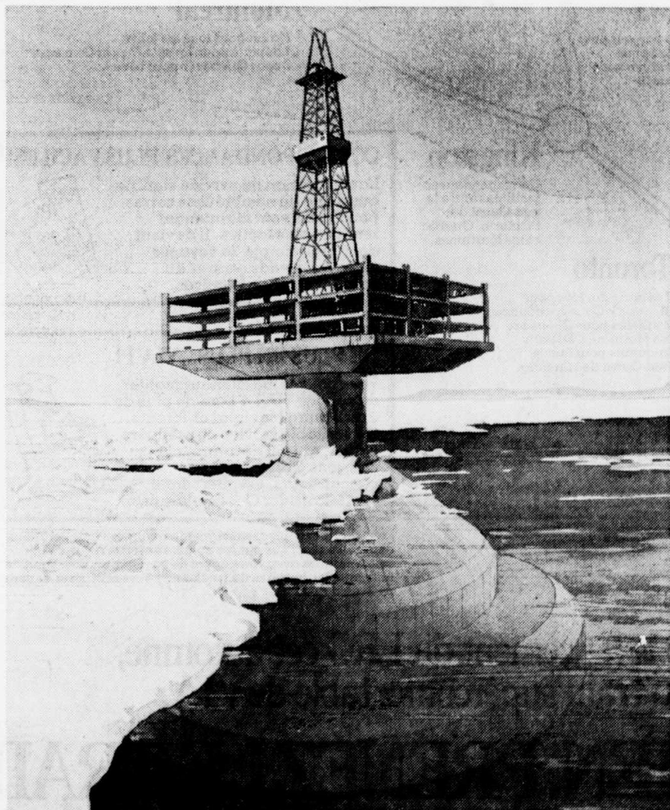
Cette "pyramide circulaire" est un des premiers concepts envisagés pour extraire sans danger le pétrole contenu sous la mer de Beaufort. D'autres concepts encore plus audacieux pour faire face au défi que posent les glaces de l'océan Arctique sont à l'étude chez Gulf. Quelle que soit la solution finale, des centaines de millions de dollars seront investis avant que le premier baril de pétrole brut ne parvienne au consommateur.
