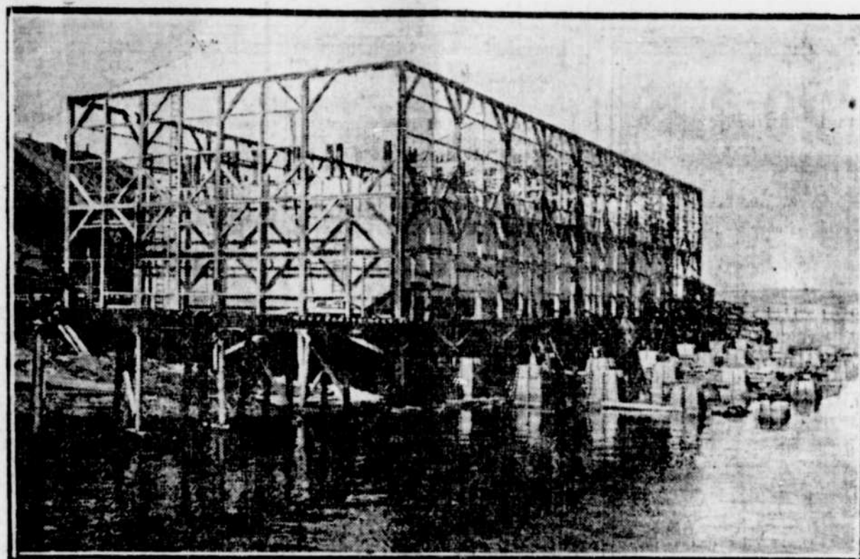
L'ENORME CAISSON, (vue du fleuve), que sont à construire, à Sillery, M. M. Davis. — Ce caisson sera lancé à la fin du mois, puis parachuté dans l'anse de Sillery, avant d'être mis en place, sur la rive nord du fleuve. Ce caisson servira d'appui au pilier nord du pont de Québec.
