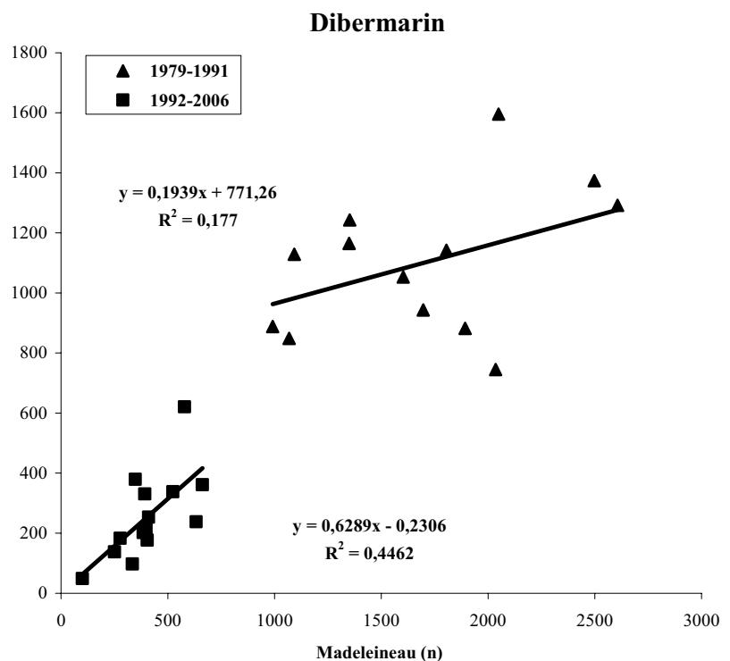
Figure 16. Relation entre la montaison de madeleineaux et celle des grands saumons un an plus tard, incluant la pêche commerciale, rivière de la Trinité, 1979-2006.
