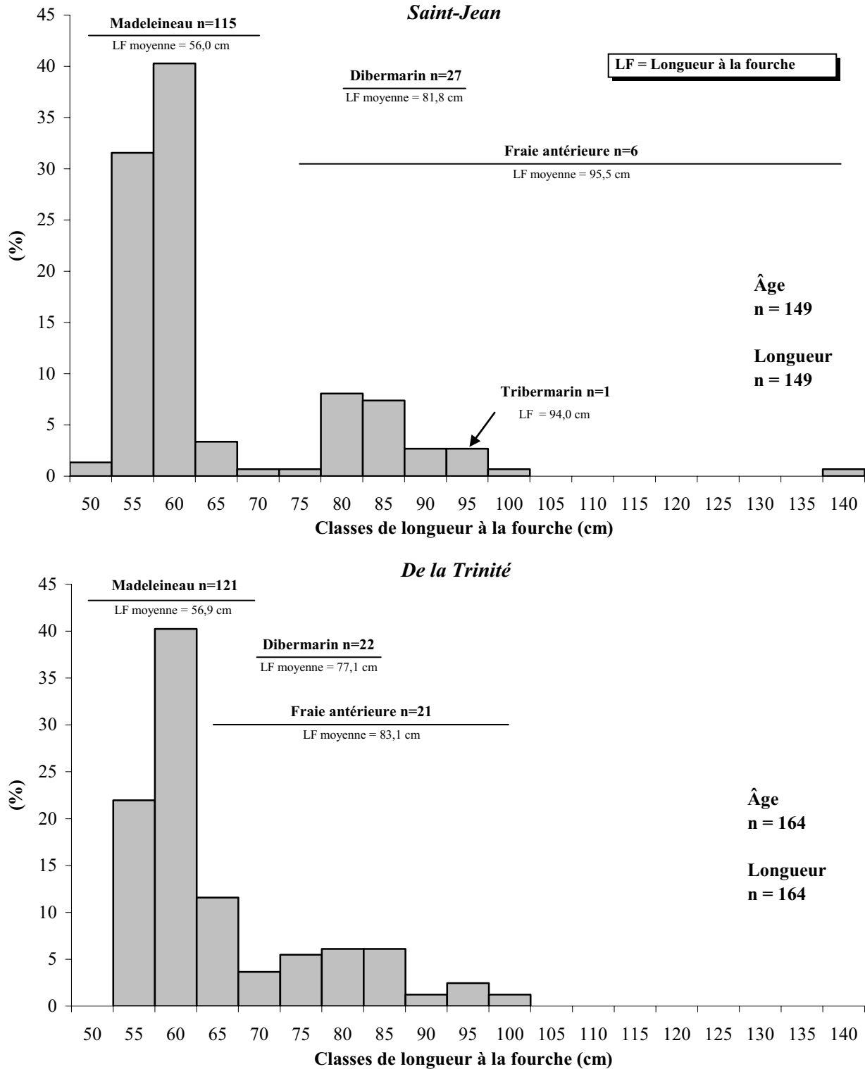
Figure 10. Fréquence de longueur et intervalles de classes de longueur en fonction de l'âge des saumons adultes échantillonnés, rivière Saint-Jean et rivière de la Trinité, 2006.
