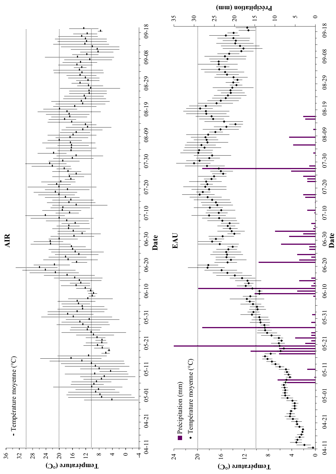
Figure 3. Précipitation et température journalière de l'air et de l'eau, rivière Saint-Jean, 2006.
