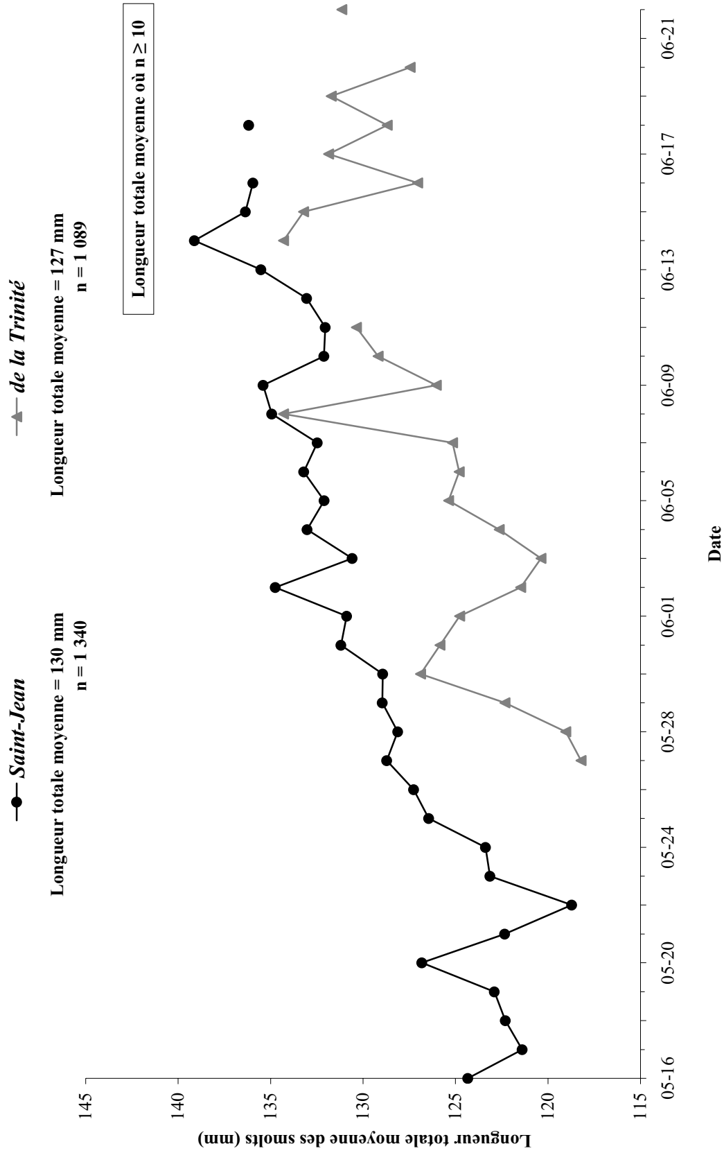
Figure 7. Comparaison de la longueur totale moyenne journalière des smolts, rivière Saint-Jean et rivière de la Trinité, 2006.
