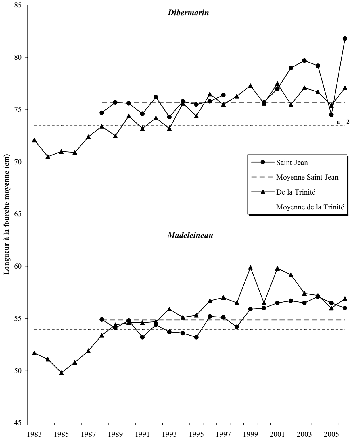
Figure 12. Longueur à la fourche moyenne des saumons des rivières Saint-Jean et de la Trinité, 1983-2006.
