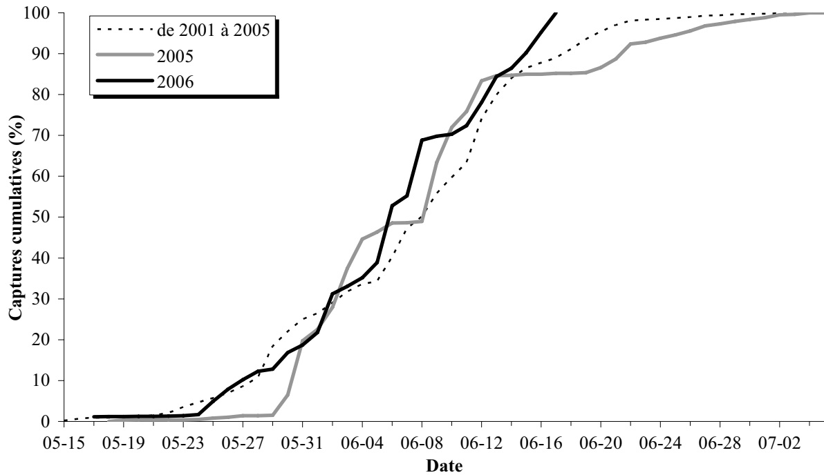
Figure 17. Anguilles capturées dans la trappe rotative, rivière Saint-Jean, 2001-2006.
