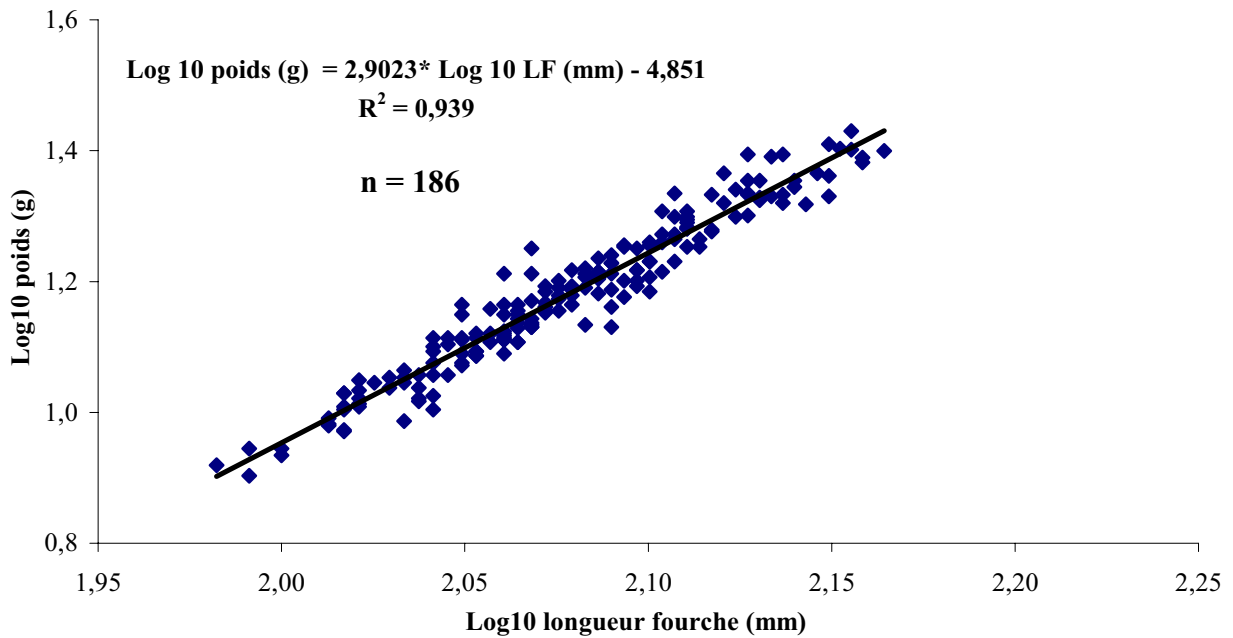
Figure 9. Relation longueur-poids des smolts, rivière Saint-Jean et rivière de la Trinité, 2006.
