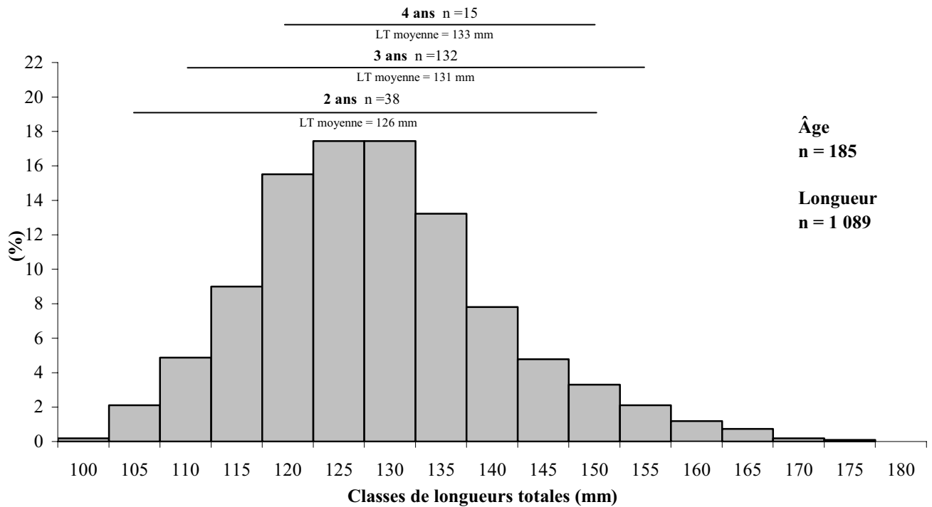
Figure 8. Fréquence de longueur des smolts mesurés vivants et intervalles de classes de longueur en fonction de l'âge des smolts collectionnés, rivières Saint-Jean et de la Trinité, 2006.
