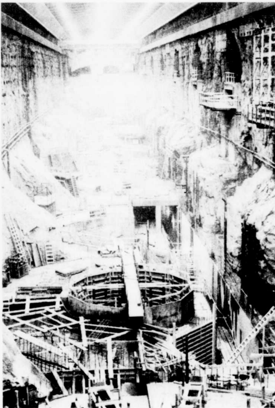
Dans la chambre des turbines, les travaux progressent surtout auprès de quatre groupes turbine-alternateur que la SEBJ espère mettre en marche à l'automne 1979.
