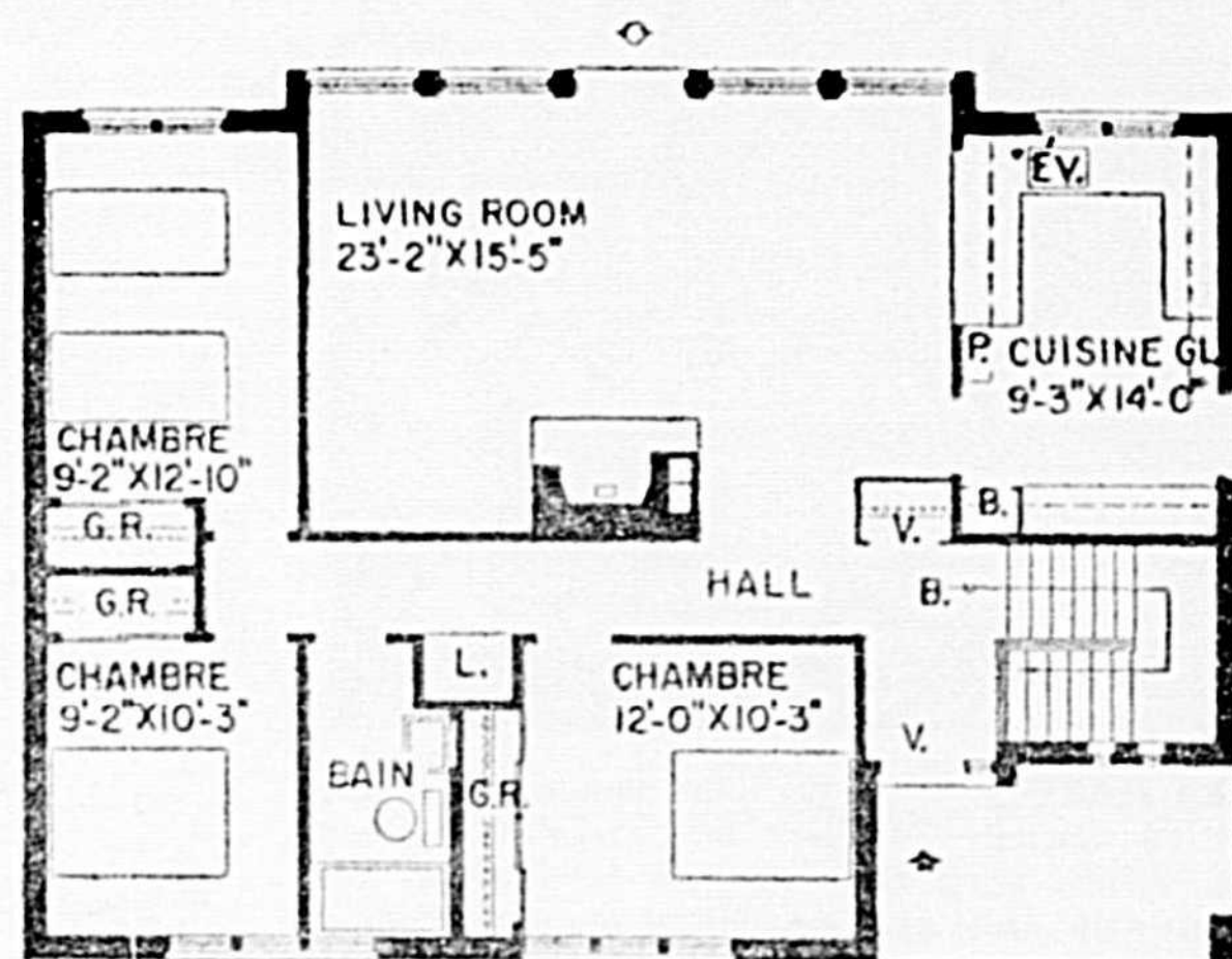
MODÈLE 273: L'architecte Dennis Peters, de Oakville, a dessiné le modèle de ce bungalow de trois chambres en brique massive. L'aire totale de parquet de la maison est de 44 pieds sur 29 pieds 9 pouces. On peut se procurer les épures de ce plan au prix minimum à la Société centrale d'hypothèques et de logement.
