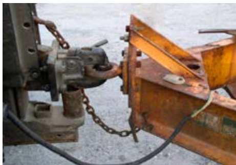
FIGURE 3 | Crochet et anneau
