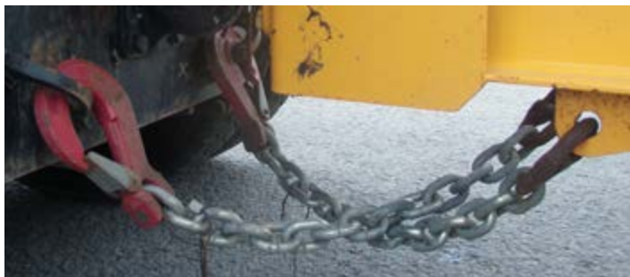
FIGURE 15 | Attaches de sûreté et leurs raccords
