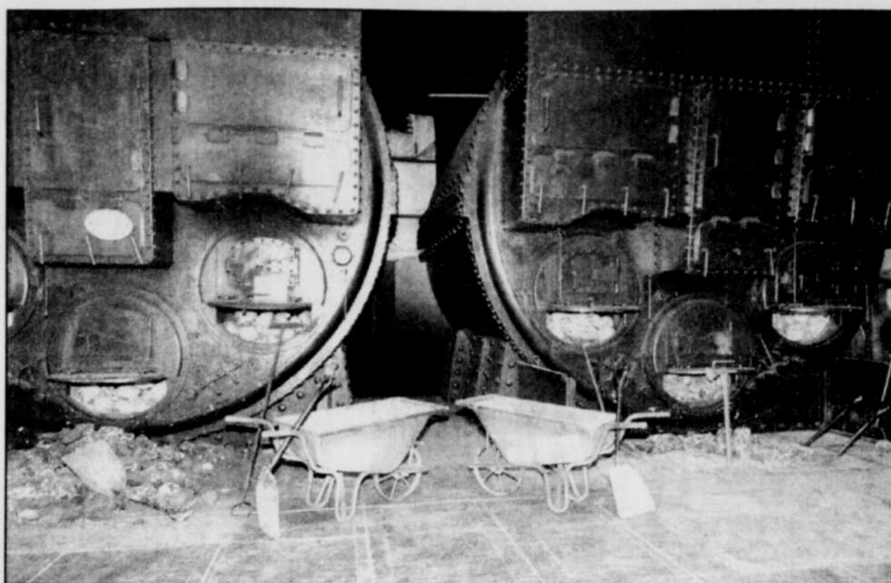
La salle des chaudières fait maintenant partie du «musée Titanic».
