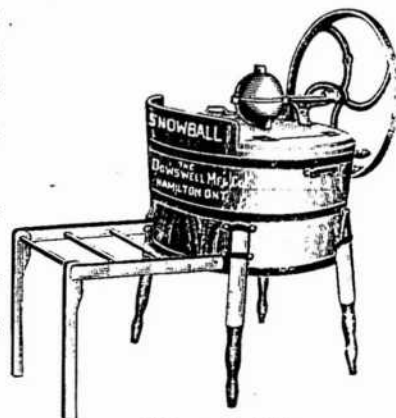
"Snowball"
