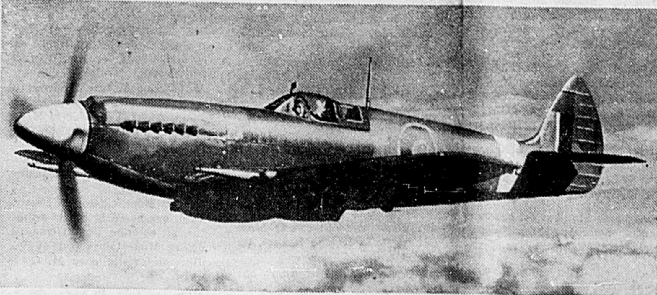
Photographie du dernier modèle du fameux Spitfire de la R.A.F. Le Spitfire modèle XII avec le moteur Rolls Royce Griffon. Notons en particulier les ailes abattues, pour combat à basse altitude, le nouveau gouvernail à pointe et le nez à forme nouvelle qui enveloppe le moteur.
