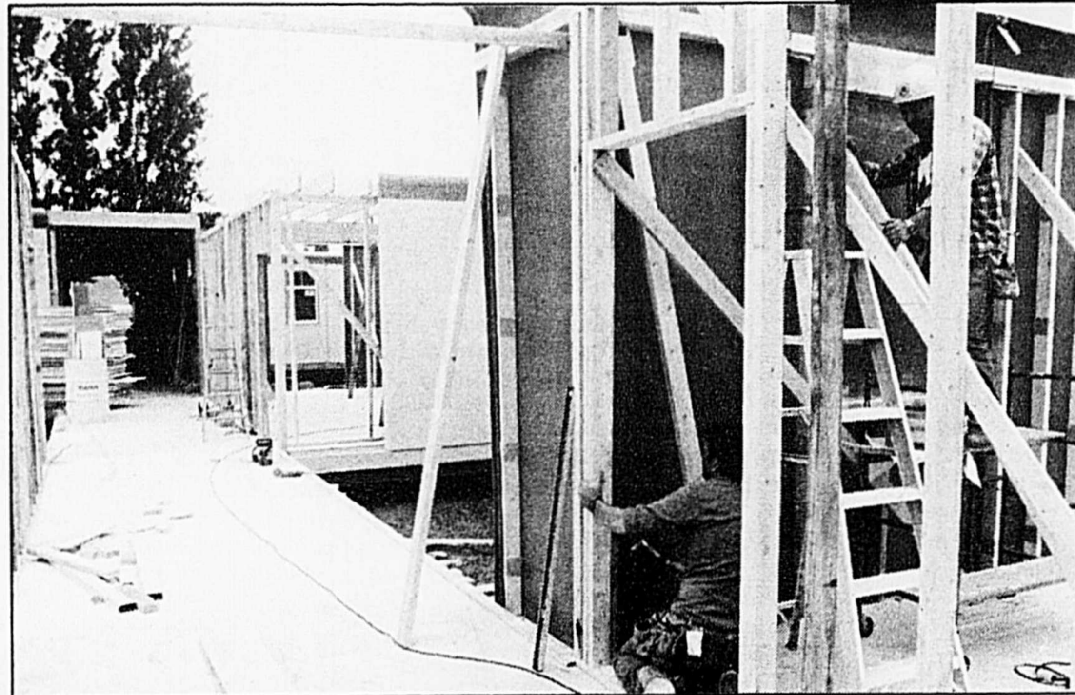
Les travaux d'assemblage se font sur place plutôt qu'en usine où les ouvriers ne pourraient travailler qu'à un maximum de 3 modules à la fois. Sauf les fenêtres, il n'y a pas de travaux de peinture prévus, les murs étant recouverts de gypse ('gyproc') pré-traité.
