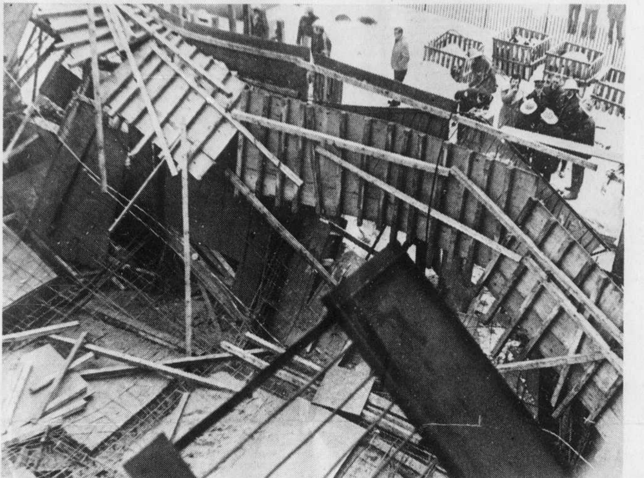
Cinq ouvriers de la compagnie De Mix Lt  e ont subi des blessures l  g res ou des fractures, hier    Longueuil lorsque des coffrages se sont effondr  s, les ensevelissant dans le b ton fluide. L'incident est survenu juste en face de la station de m tro, sur la rue Dasigny, l   o   l'on construit un  difice en hauteur.
