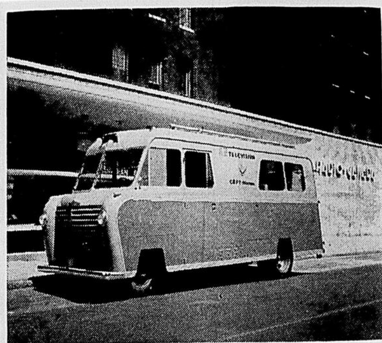
● LE CAR DE REPORTAGE de CBFT est en quelque sorte une cabine de contrôle sur roues qui se sert de toute la métropole comme studio. Son équipage formé de 10 hommes, trois caméras et un émetteur de micro-ondes, peut transmettre des reportages en direct dans un rayon de vingt milles de la tour du mont Royal. Il n'existe que deux cars du genre au Canada, l'autre appartenant au poste CBLT de Radio-Canada à Toronto. Chacun a coûté environ $100,000.
