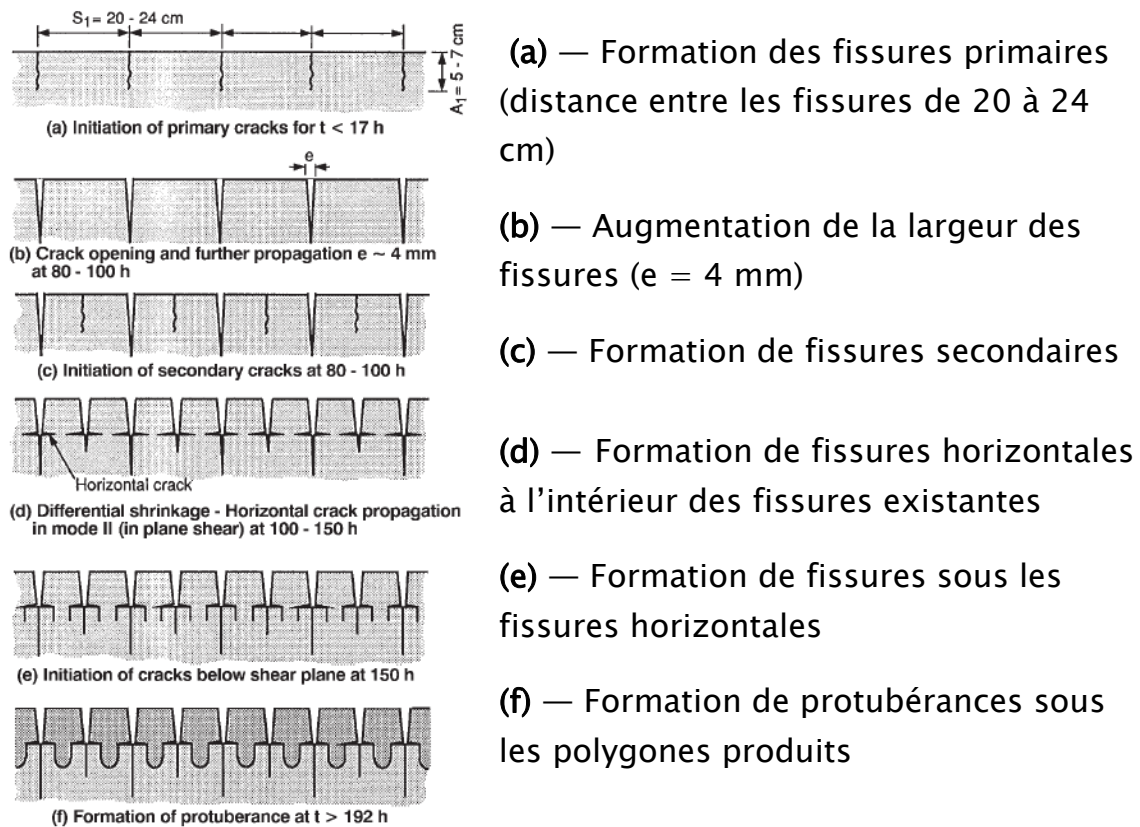
Figure 3. Étapes de fissuration d'une argile St-Alban intacte (Konrad et Ayad, 1997).
