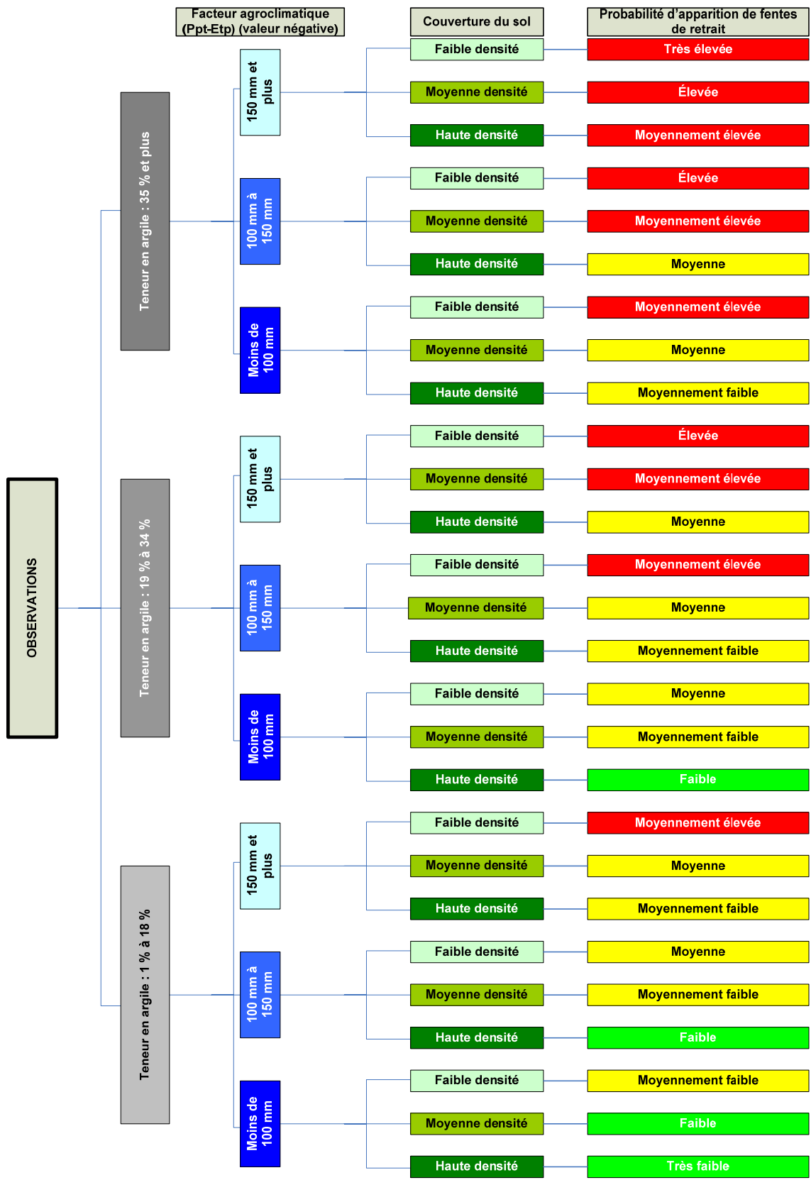
Figure 5. Schématisation du risque d'apparition de fentes de retrait.
