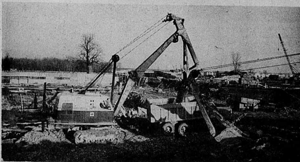
Les travaux de construction de l'Institut de Recherche de l'Hydro-Québec sont en cours à 18 milles au sud-est de Montréal, près du poste à 735 kV de Boucherville.
