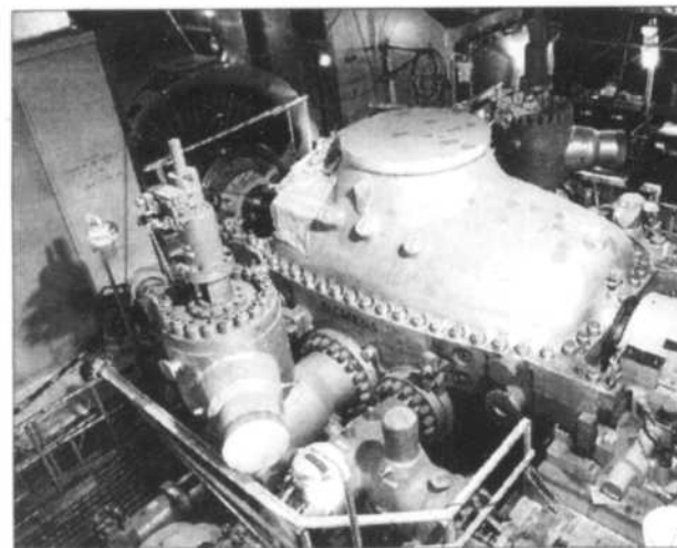
On est ici au cœur de la centrale de cogénération de Bécancour. Cette centrale produira de la vapeur et environ 4,5 térawatts d'énergie par année, soit un volume suffisant pour répondre aux besoins de 500 000 foyers.
