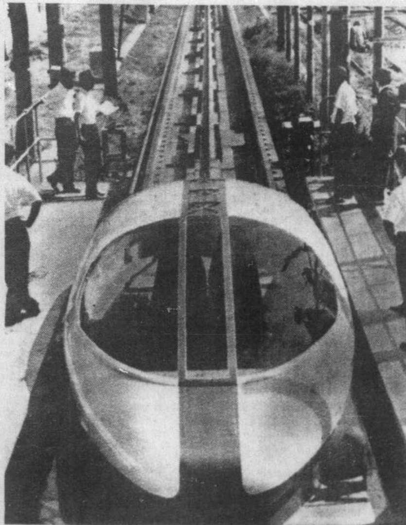
Regardez bien! Il s'agit du train des années 1980. Des techniciens de l'Institut de recherche technique de Tokyo procèdent ici, le long d'un rail d'essai, à des tests sur un wagon en forme d'oeuf qui ferait partie d'un train capable de circuler à plus de 300 milles à l'heure. Le train, mû par des moteurs à induction linéaire, se déplace à 2 1/2 pouces au-dessus du sol. (Téléphoto AP)
