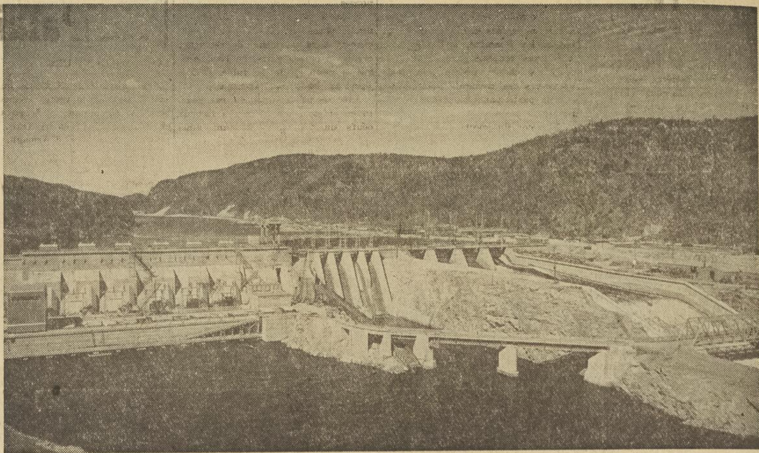
La nouvelle centrale de la compagnie Shawinigan Water and Power, au rapide Beaumont sur le haut St-Maurice, dont la puissance sera de 246,200 kilowatts. De gauche à droite: le barrage principal et la centrale, l'ouvrage de régularisation, le déversoir et l'évacuateur de crues.
