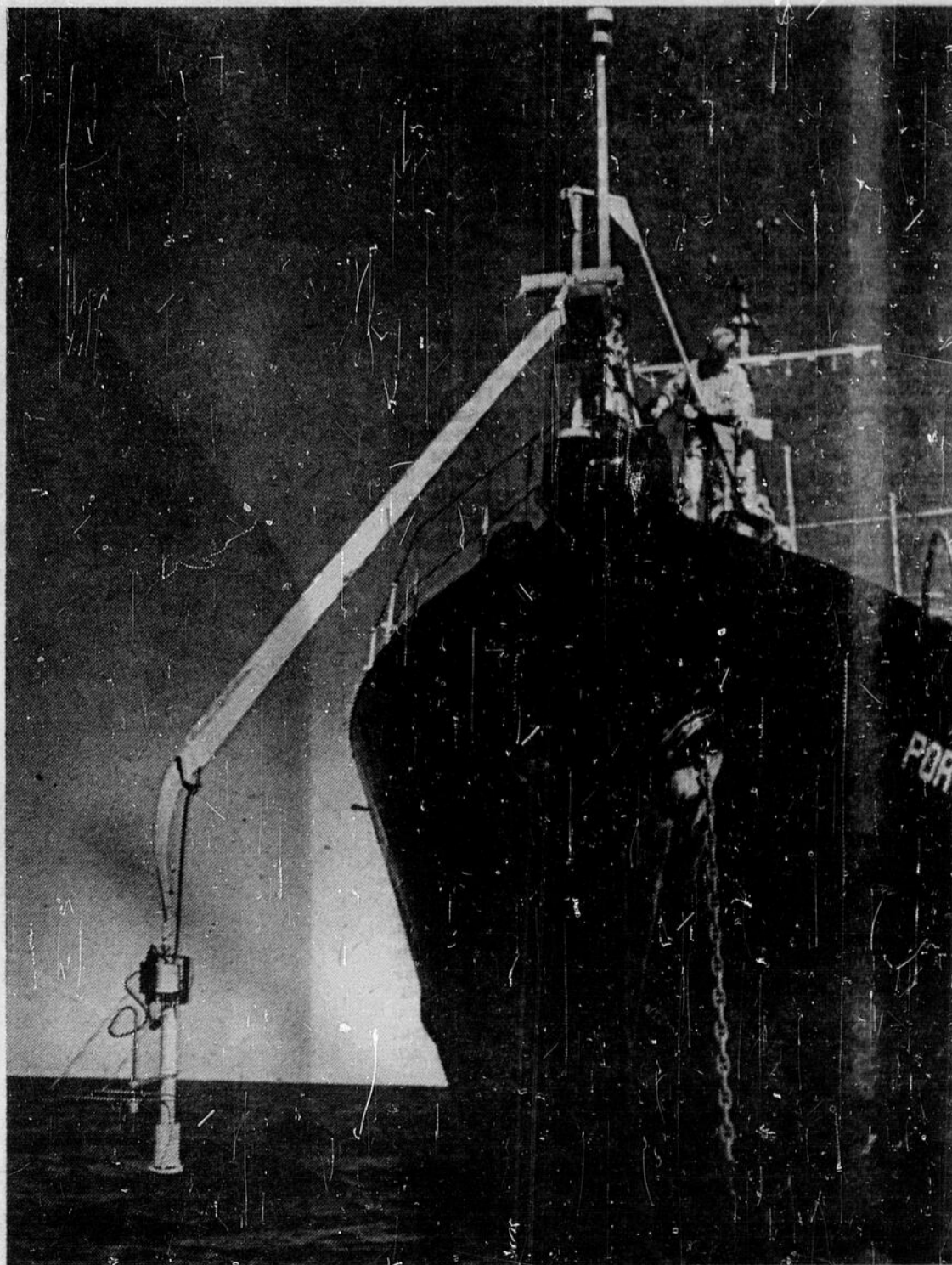
C'est à l'aide d'un treuil bien particulier, auquel on a fixé des instruments, que l'on obtient des données sur les conditions atmosphériques variant du niveau de l'eau à quarante-pieds dans les airs.
