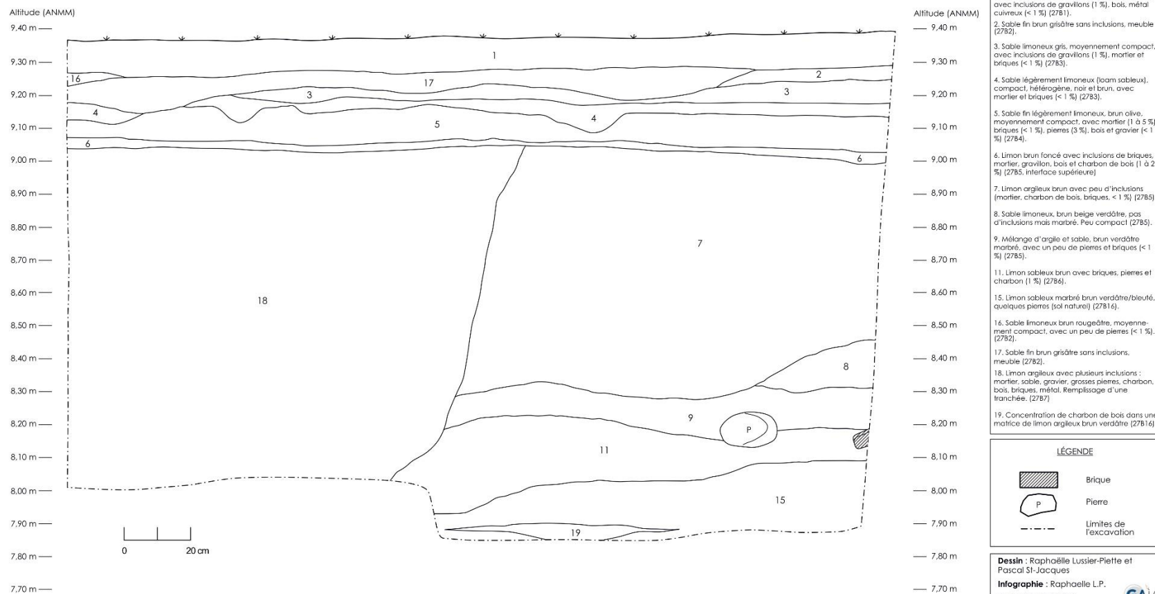
Figure 71 : Coupe stratigraphique de la paroi nord de la sous-opération 27B.
