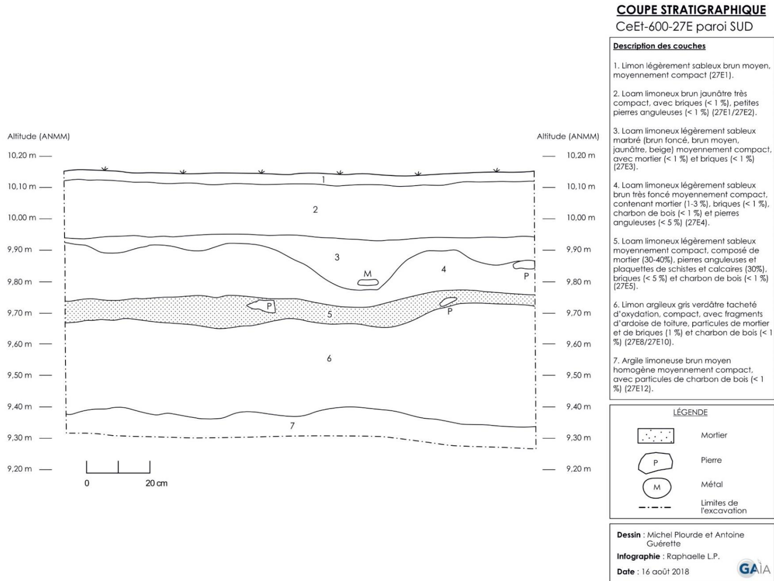
Figure 81 : Coupe stratigraphique de la paroi sud de la sous-opération 27E.
