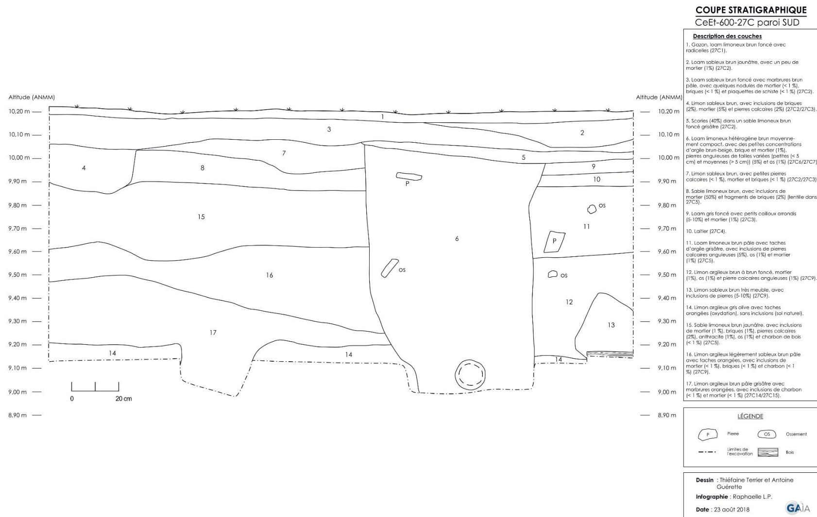
Figure 78 : Coupe stratigraphique de la paroi sud de la sous-opération 27C.
