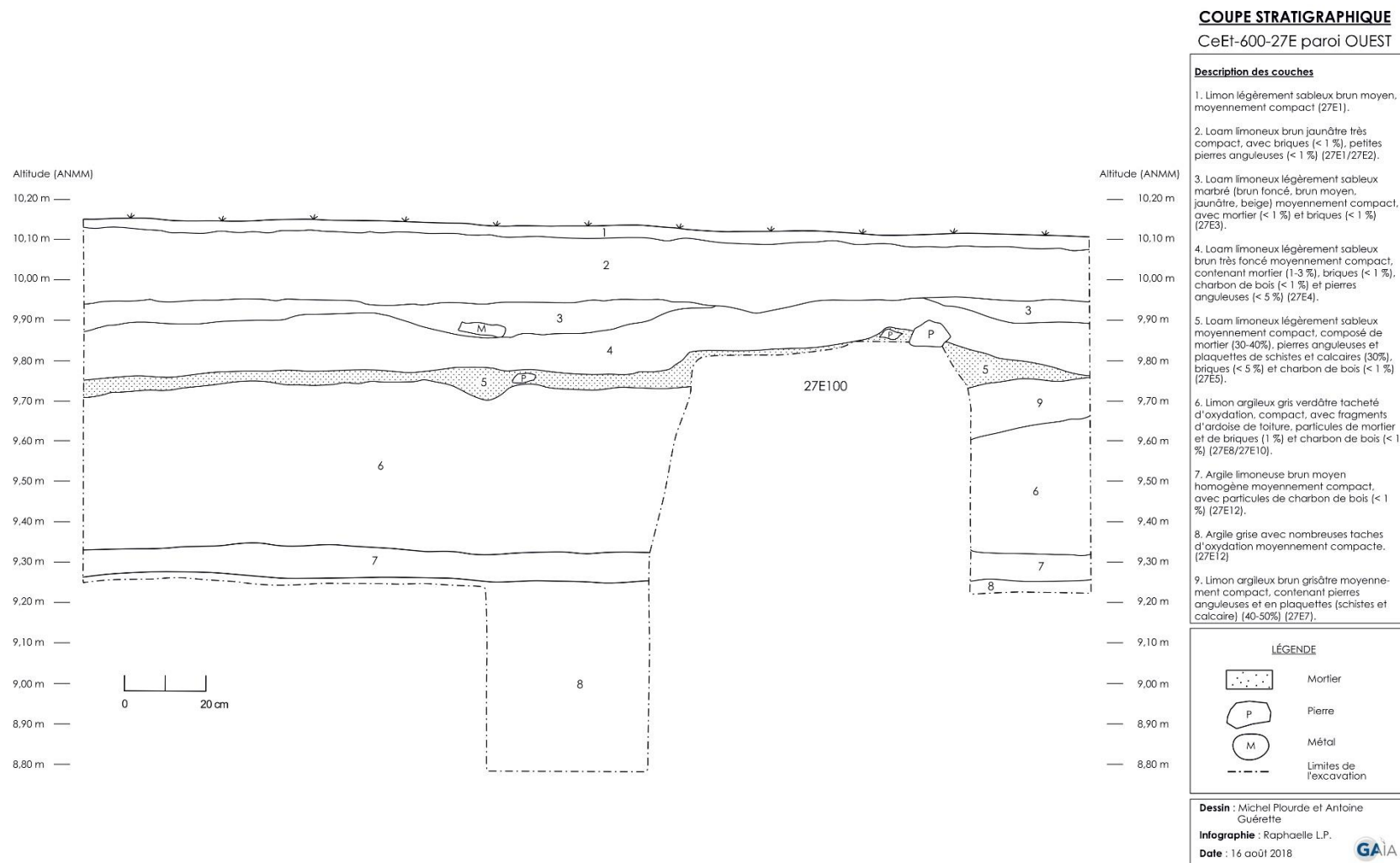
Figure 80 : Coupe stratigraphique de la paroi ouest de la sous-opération 27E.
