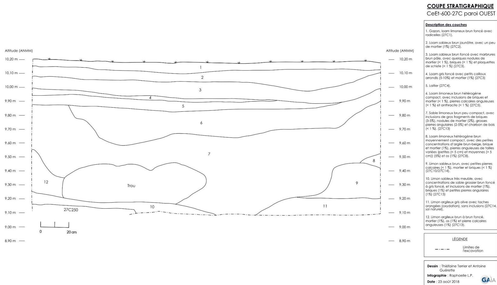
Figure 77 : Coupe stratigraphique de la paroi ouest de la sous-opération 27C.
