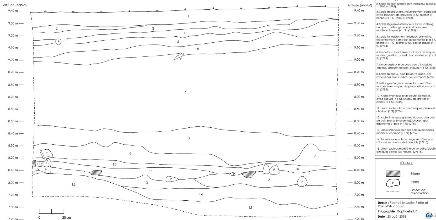
Figure 70 : Coupe stratigraphique de la paroi est de la sous-opération 27B.
