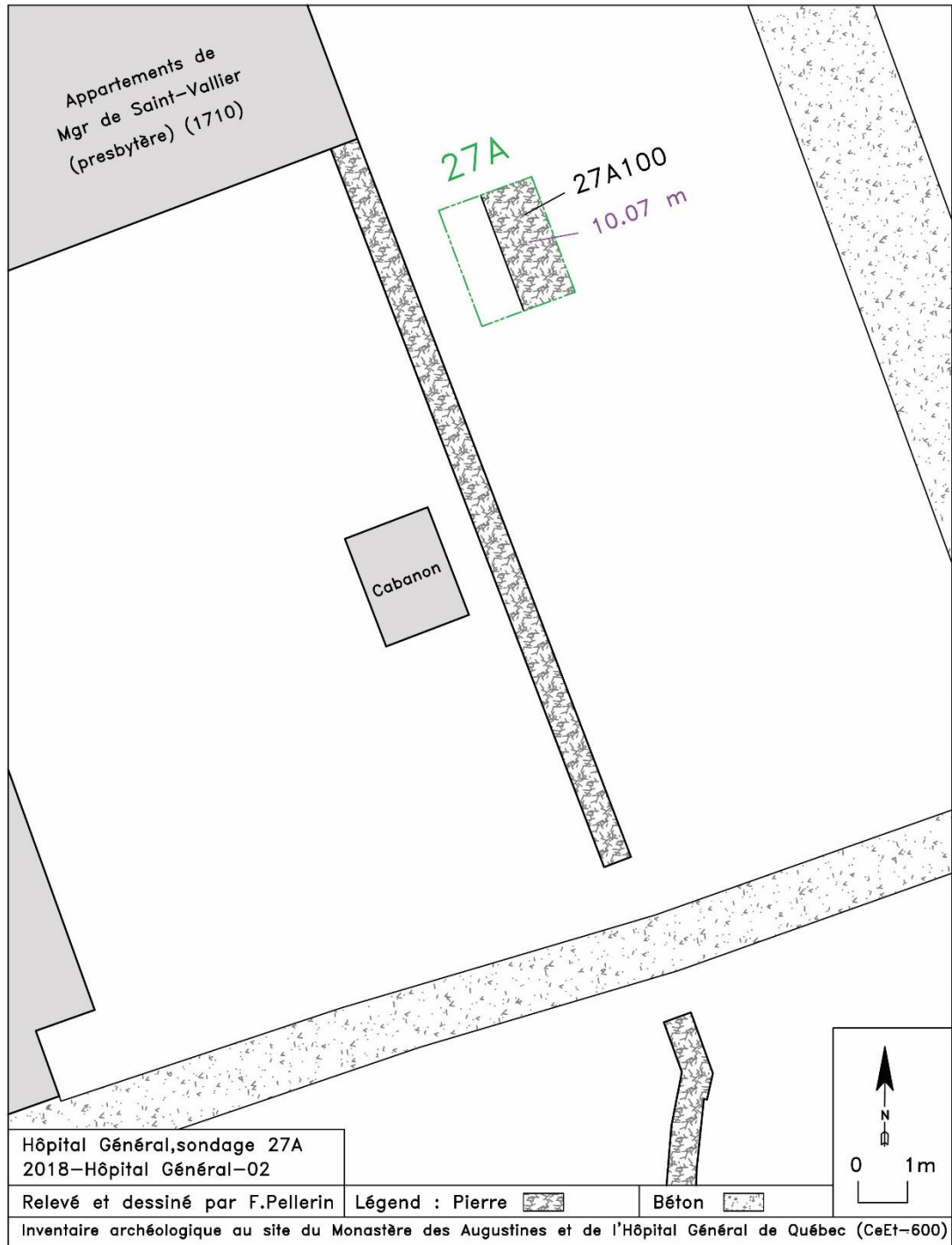
Figure 66 : Plan d'intervention de la sous-opération 27A.
