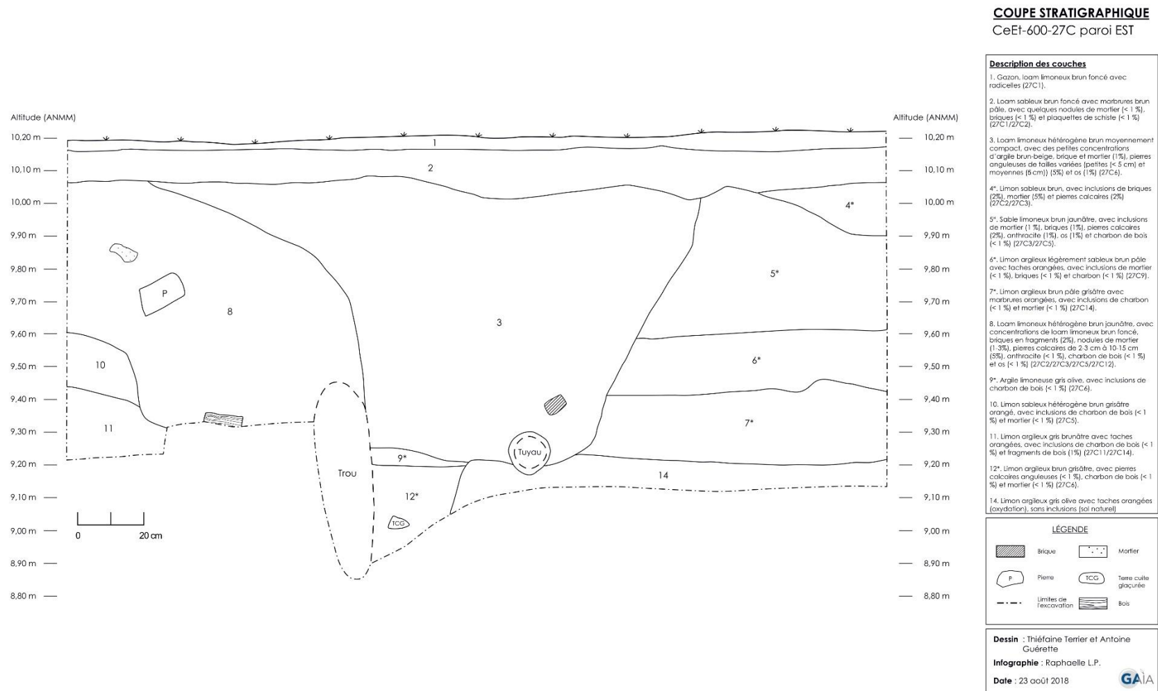
Figure 75 : Coupe stratigraphique de la paroi est de la sous-opération 27C.
