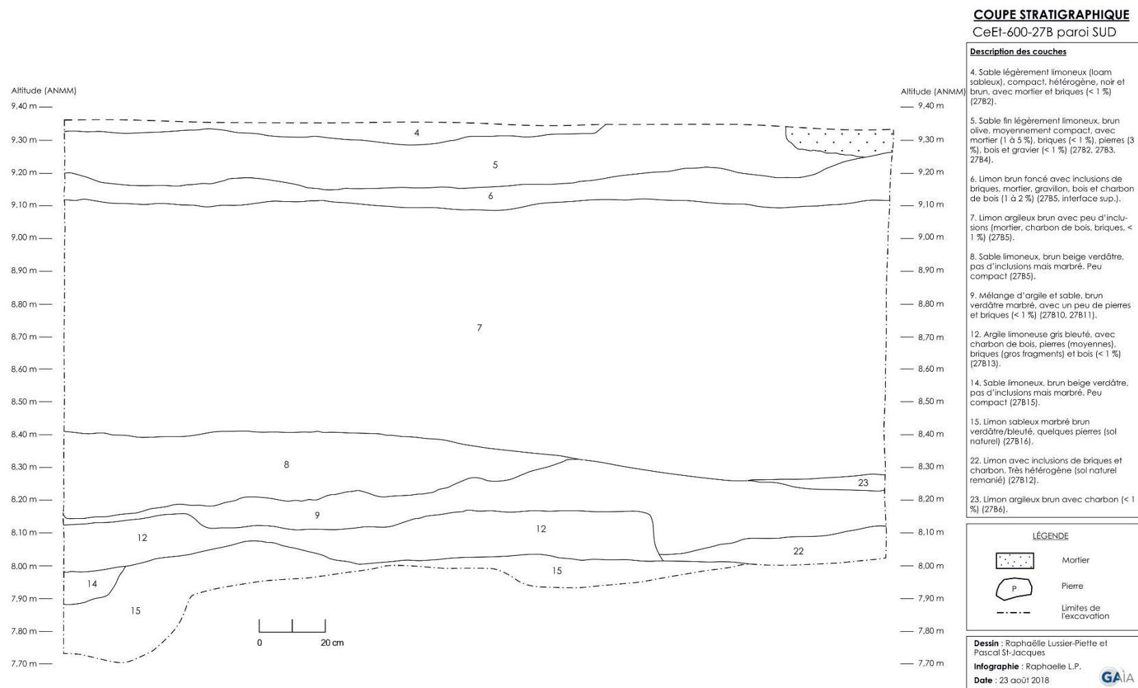
Figure 72 : Coupe stratigraphique de la paroi sud de la sous-opération 27B.
