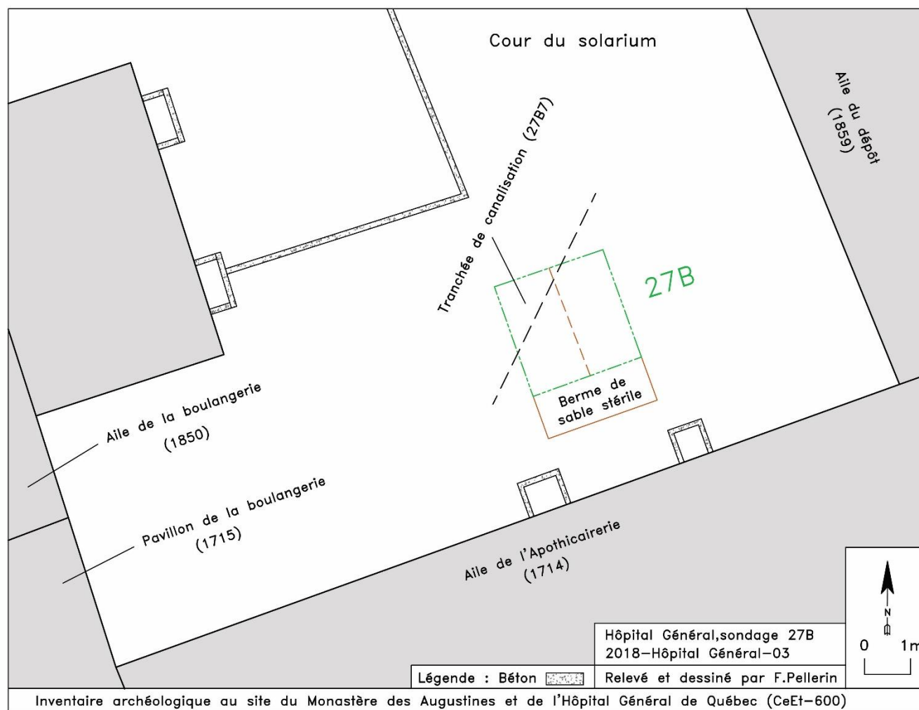
Figure 17 : Localisation de la sous-opération 27B à l'intérieur de la cour du solarium.
