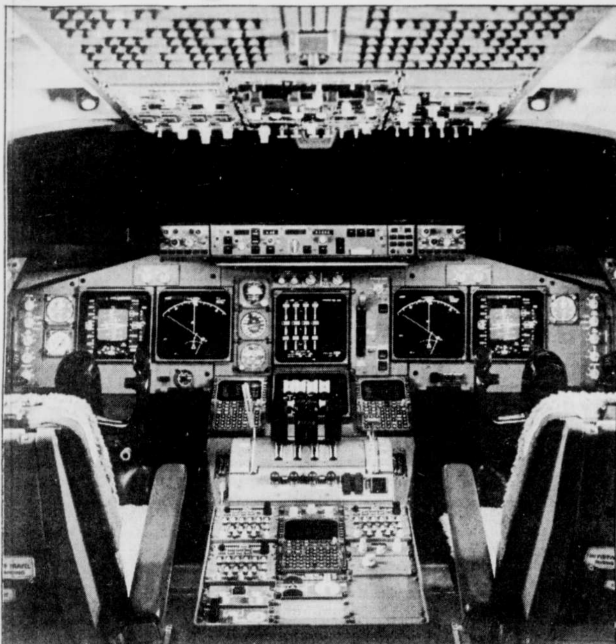
Le poste de pilotage du nouveau 747-400 de Boeing intègre de nombreux écrans sur lesquels sont affichées les fonctions de vol, des moteurs, de navigation et d'alerte de l'équipage, bref on a réduit le nombre de lampes, de cadrans, de jauges et d'interrupteurs.
