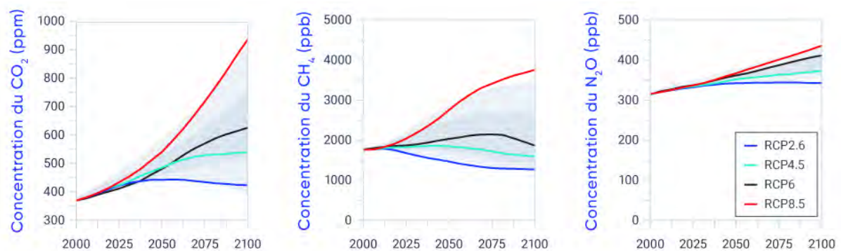
Figure 1 Concentrations de \text{CO}_2 en fonction des scénarios climatiques du GIEC
