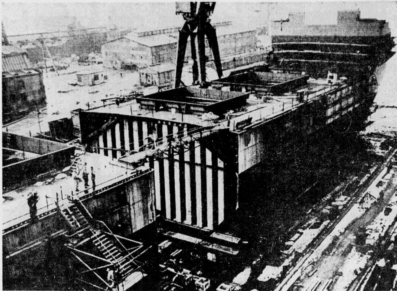
UNE RALLONGE POUR LE NAVIRE — Ce navire en construction dans un chantier naval de Hambourg était prêt pour le lancement lorsqu'on décida au dernier moment de le rallonger de 15 mètres! C'est la première fois en Allemagne que l'on
