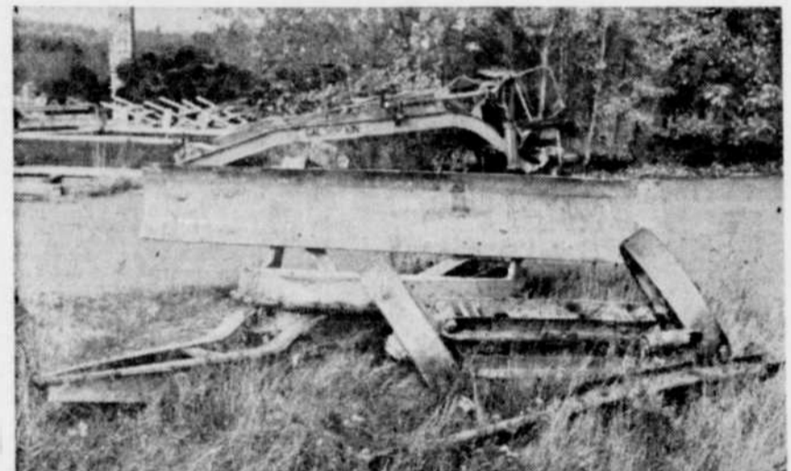
Sous la violence du choc, une section du bélier mécanique a été projetée à plusieurs pieds de la voie ferrée.
