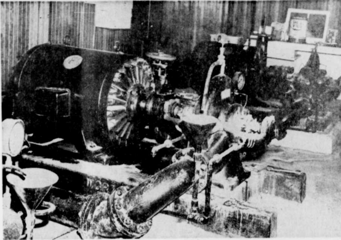
Usine de pompage. — L'eau provenant du puits artésien et des sources naturelles, qui alimentent le réseau d'aqueduc municipal, est premièrement déversée dans un réservoir intermédiaire pour ensuite être dirigée vers le réservoir souterrain d'une capacité de deux millions de gallons. Sur cette photo nous voyons deux des trois moteurs de l'usine de pompage, dont la capacité est de 1,750 gallons à la minute. (Photo Ross, Coaticook)
