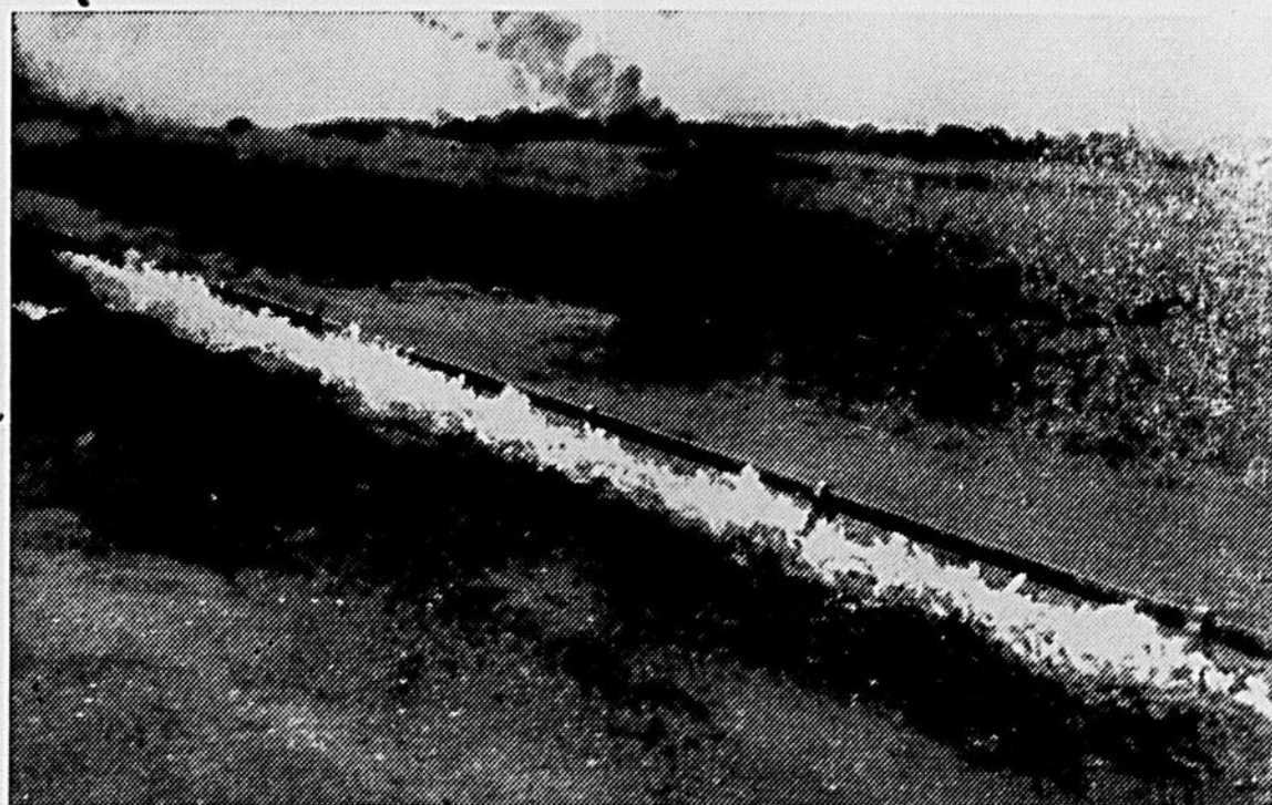
Voici l'une des premières photographies officielles d'une opération de dispersion artificielle du brouillard, sur un aérodrome de la R.A.F. L'appareil fournit la chaleur nécessaire à une double rangée de brûleurs, installés de part et d'autre de la piste. Cet appareil appelé FIDO (nom formé avec les initiales de "Fog Investigation Dispersion Operations") est une invention de guerre. La photo a été prise au moment où les flammes commencent à courir le long de la rangée de brûleurs.
