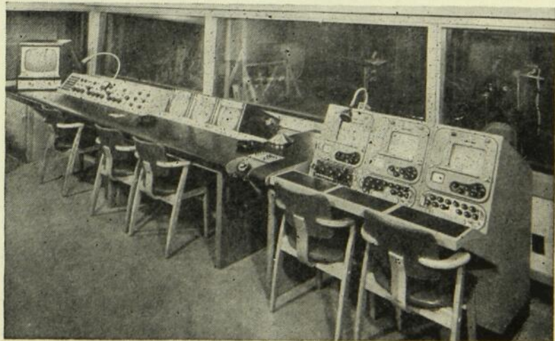
La salle de contrôle du studio 41, le moins grand des deux studios de télévision qui sont logés derrière l'édifice Radio-Canada. On voit, à gauche, la console de prise de son, au centre, les écrans-viseurs du réalisateur et de son assistante et, à droite, les écrans correspondant aux caméras logées dans les studios.
